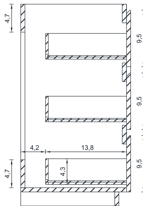
A-A SECTION
