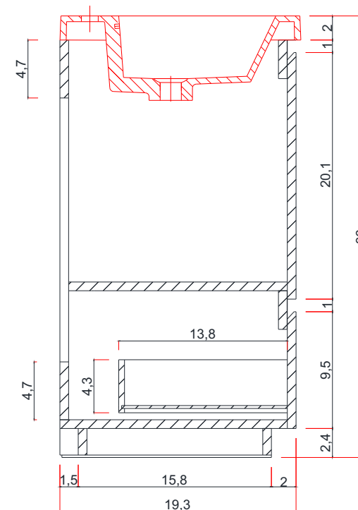
B-B KESİTİ
