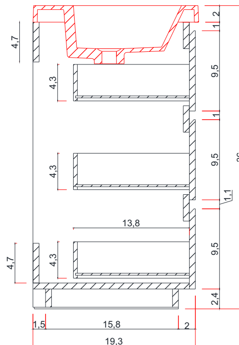
A-A KESİTİ
