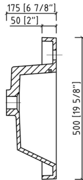
SECTION A-A
