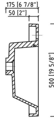
SECTION A-A
